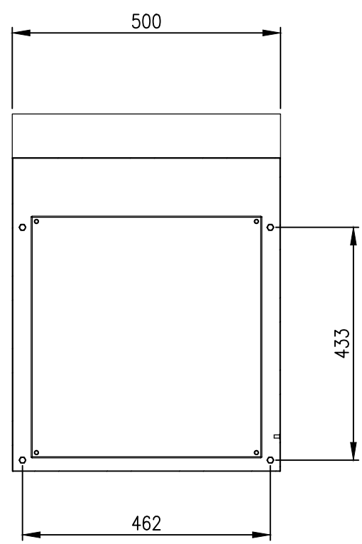
SECTION AU-AU
