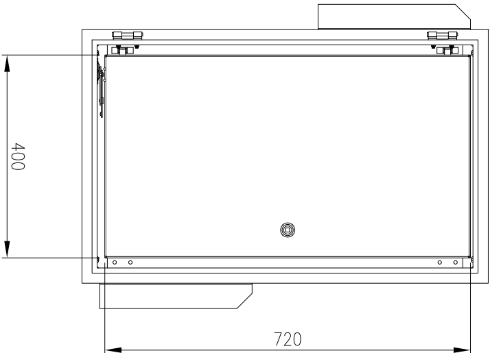
SECTION AA INNER DOOR
