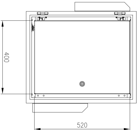
SECTION AA INNER DOOR
