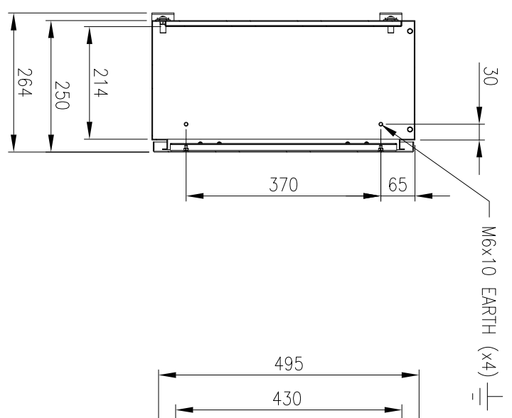
SECTION AY-AY
