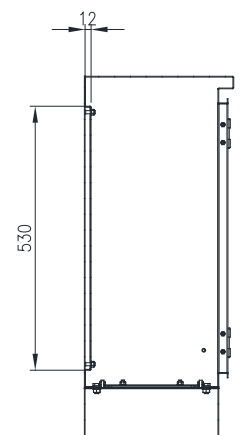
SECTION AU-AU
