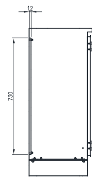
SECTION AU-AU
