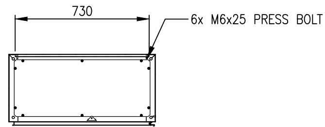
SECTION AV-AV
