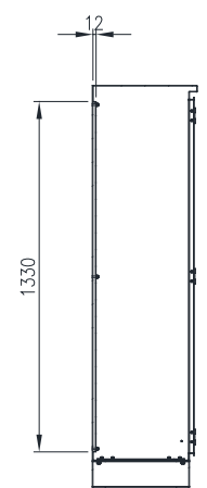
SECTION AU-AU
