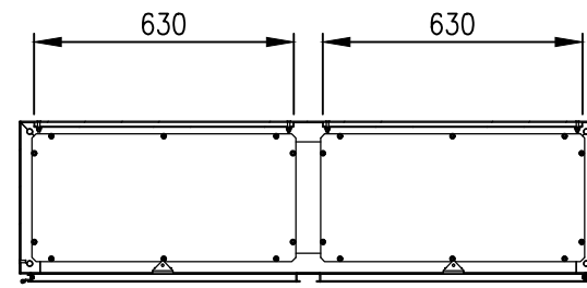
SECTION AV-AV
