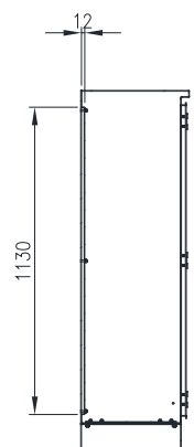
SECTION AU-AU
