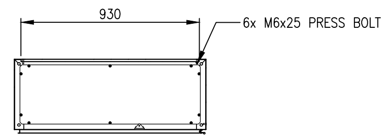
SECTION AV-AV
