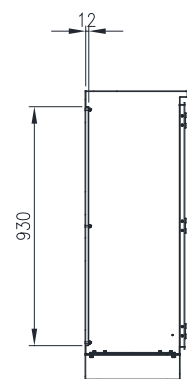
SECTION AU-AU
