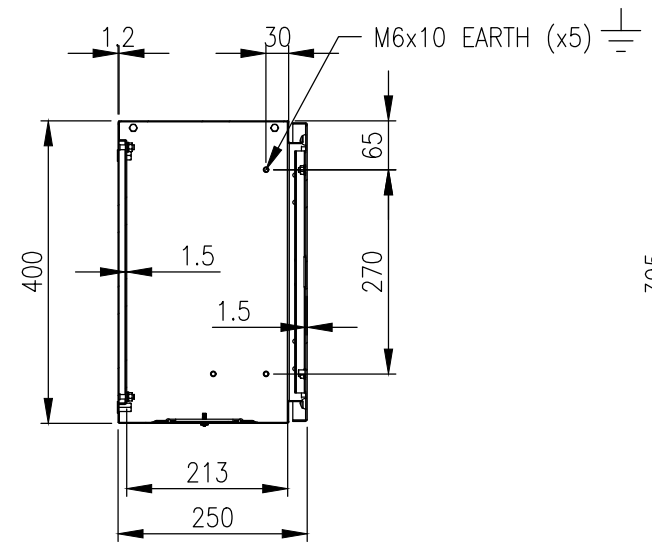
SECTION AV-AV
