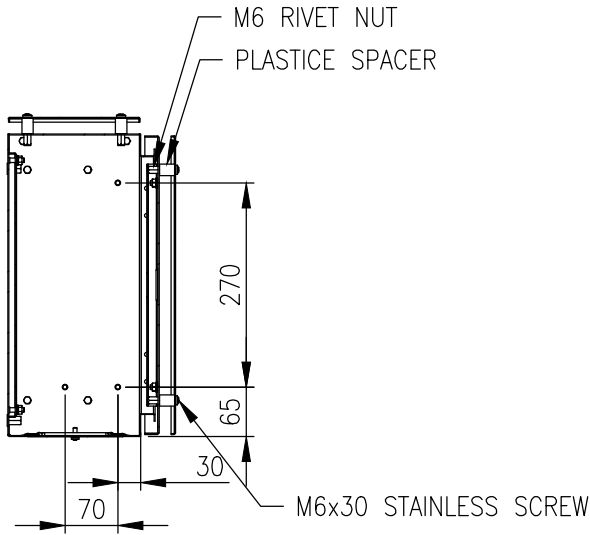
SECTION AV-AV
