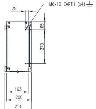
SECTION AV-AV
