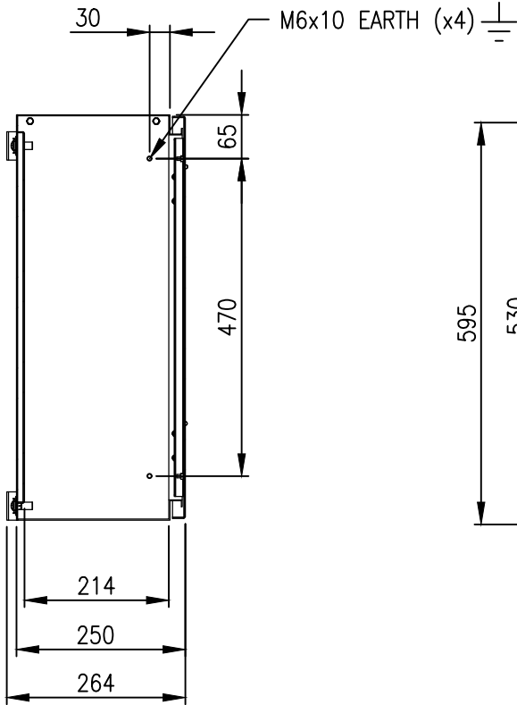
SECTION AY-AY
