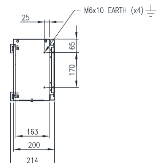
SECTION AV-AV
